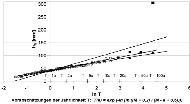
Abb. 3.1.7-1: Grafische Ermittlung der Parameter u und w auf der Basis der jährlichen Serie für Niederschlagshöhen einer Dauer von 24 Stunden am Beispiel der Station Lauenstein im Erzgebirge für 1953–2002 ( M = 50 Jahre, Quadrate), 1951 bis 2000 ( M = 50 Jahre, Dreiecke), 1951–1980 ( M = 30 Jahre, Kreise)
