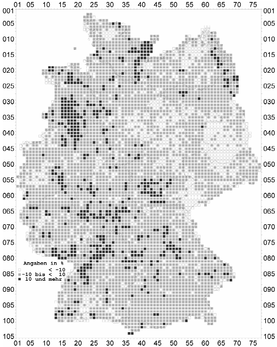
Abb. 3.1.7-3: Prozentuale Abweichungen der für den Zeitraum 1951–2000 extremwertstatistisch ermittelten Starkniederschlagshöhen von den KOSTRA-Starkniederschlagshöhen für den Zeitraum 1951–1980
