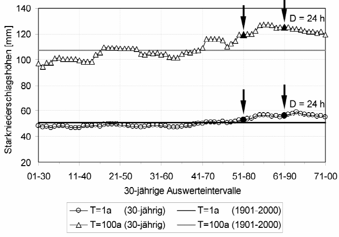
Abb. 3.1.7-2: 30-jährig gleitende Auswertungen der Station Kempten (Wst) für Starkniederschlagshöhen einer Dauer von 24 Stunden bei Wiederkehrzeiten von T = 1 a und T = 100 a im Zeitraum 1901–2000
